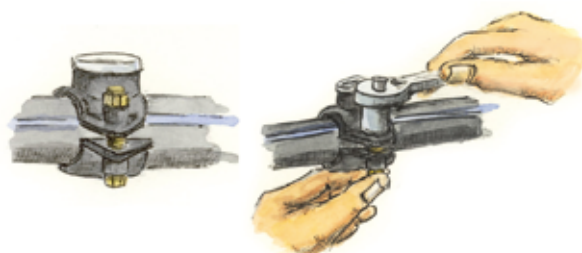
Montera bult och mutter löst för att sedan dra åt jämnt på båda sidorna av bygel
